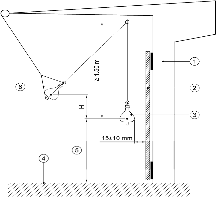
图中： H—— 跌落高度； ①—— 框架； ②—— 被测试的玻璃面板； ③—— 冲击装置； ④—— 被测试玻璃面板的参考地平面； ⑤—— 撞击点高度为1m，对于层门，该高度值见7.2.3.8； ⑥—— J2.4所述的三角钩结构。
