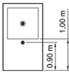
e) 在 1m 以上高度处具有玻璃面板的层门
