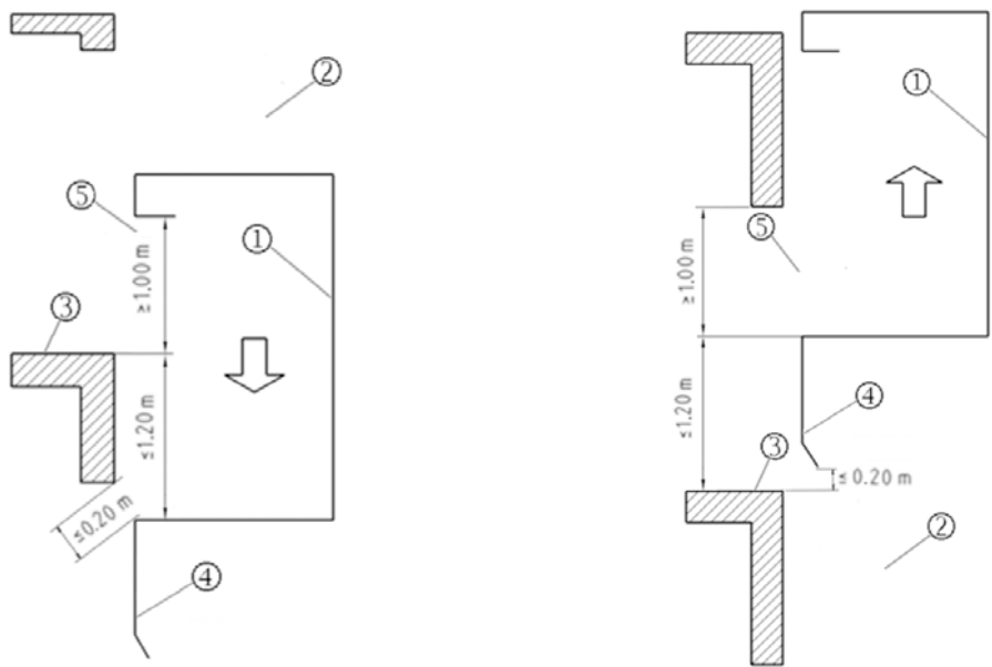
a) 向下移动
